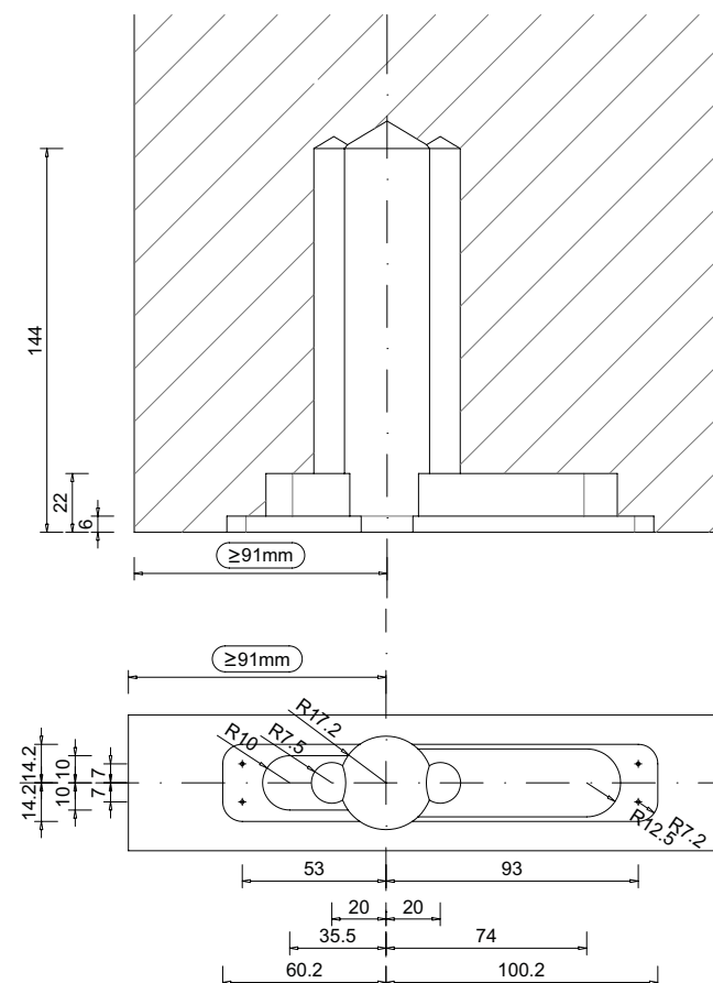
DISEGNO FRESATURA
