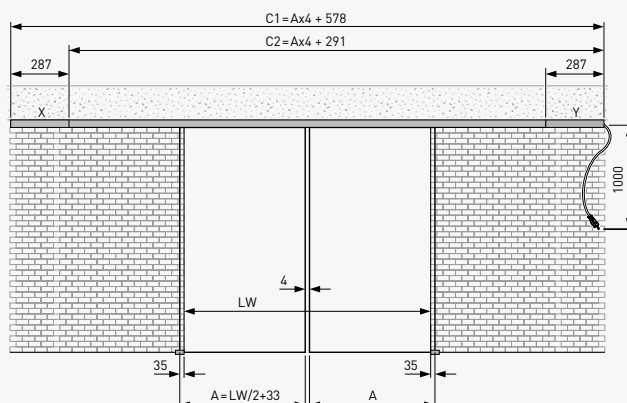
Sistemi a due ante senza anta fissa
