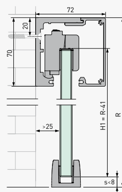
Sistemi a due ante senza anta fissa
