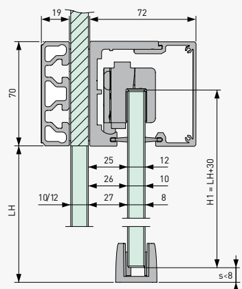
Montaggio a parete in vetro
