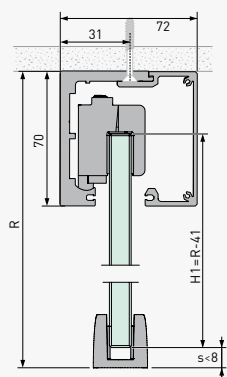
Sistemi a un'anta senza anta fissa
