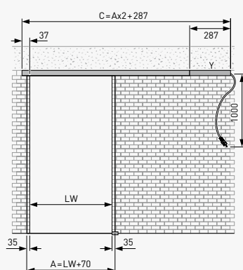
Sistemi a un'anta senza anta fissa
