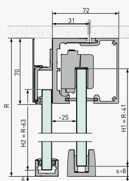
Sistemi a un'anta senza anta fissa
