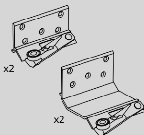
Patines inferiores Pattini inferiori Lower sliders Patins inférieurs Carros inferiores
