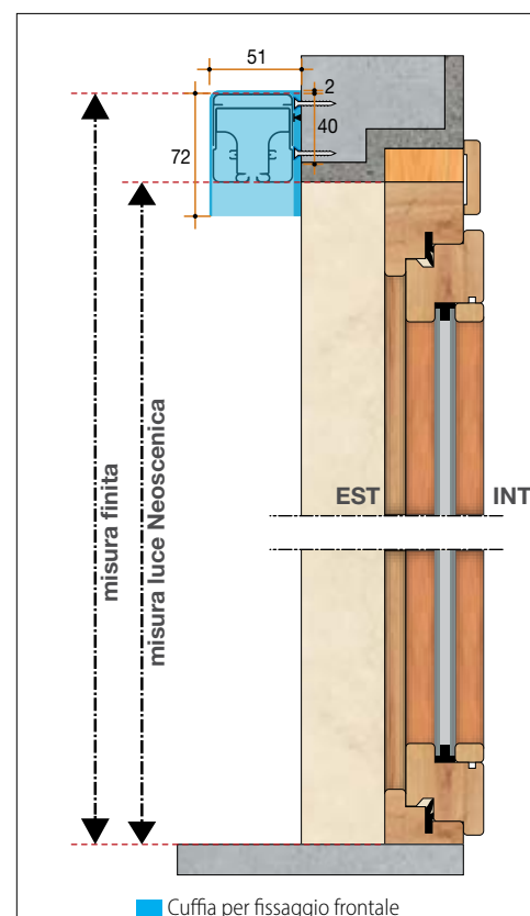
Sezione verticale
