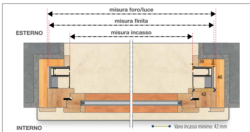
Sezione orizzontale
