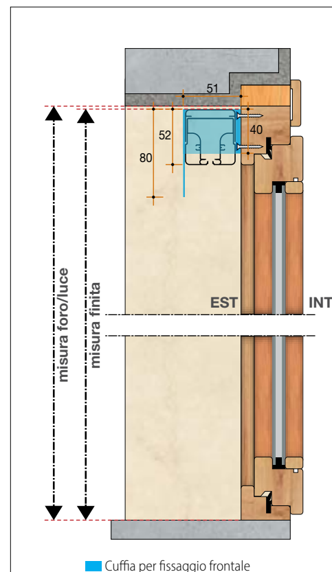
Sezione verticale
