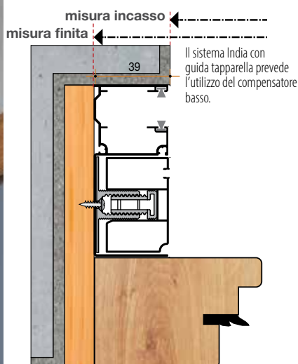
Esempio di installazione Guida Tapparella da 90mm
