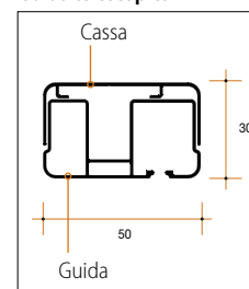
Guida telescopica
