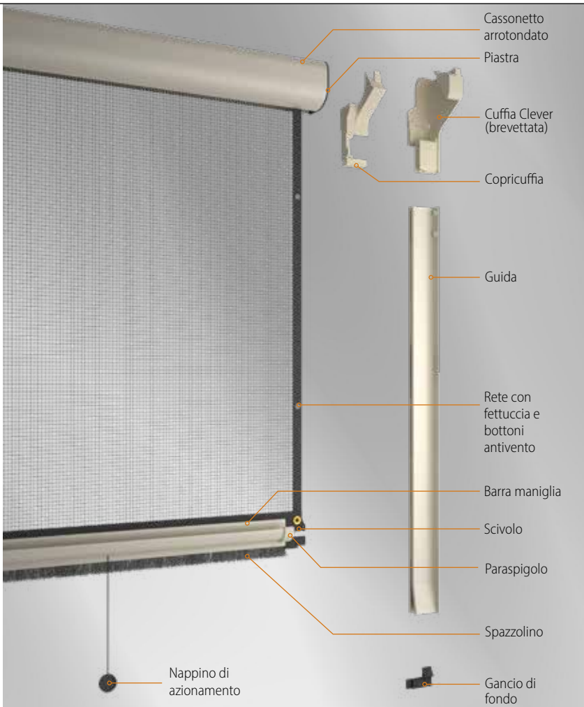
Cassonetto con barra maniglia e cuffia Clever
