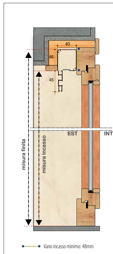
Sezione verticale
