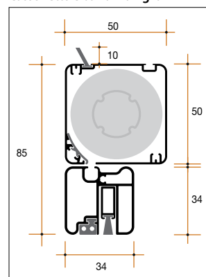
Cassonetto e barra maniglia
