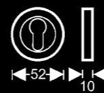
Rosette EZ 1332 - PZ Farbe: Edelstahl matt
