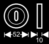
Rosette EZ 1332 - BB Farbe: Edelstahl matt
